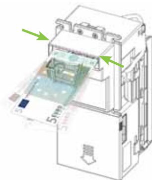
Centratura automatica Automatic centering
