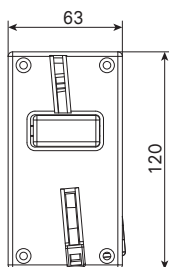
Gettoniera frontalino basso (per M20) Low front plate for Coin Selector
